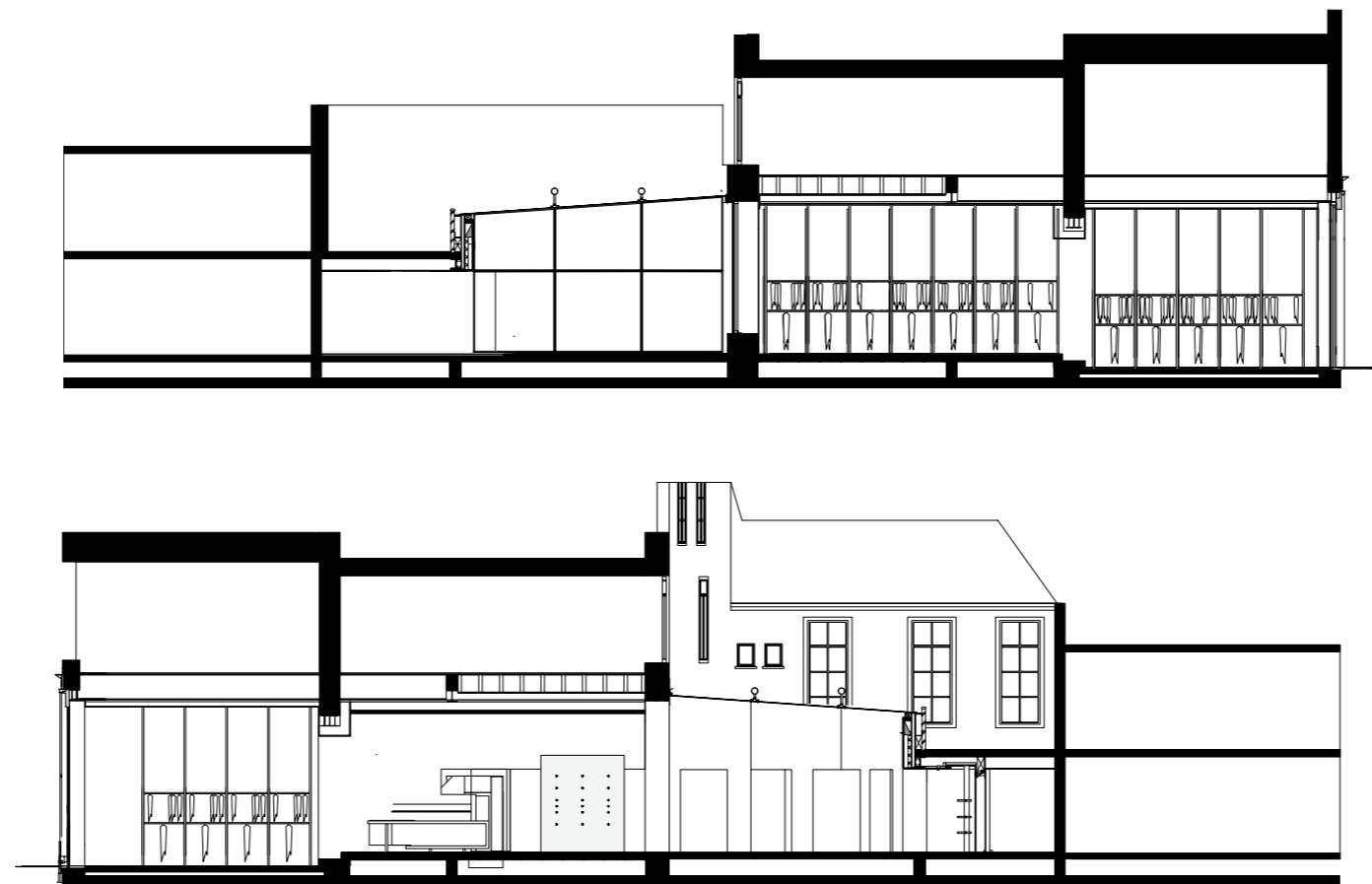
Doorsneden | sections
